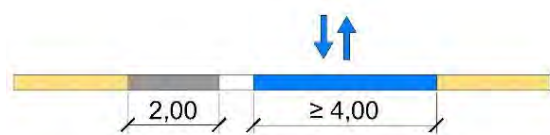
Fahrradstraße innerorts (RSW)
