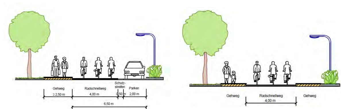
Abbildung 14: Musterquerschnitte für Fahrradstraßen (mit und ohne Parken)
