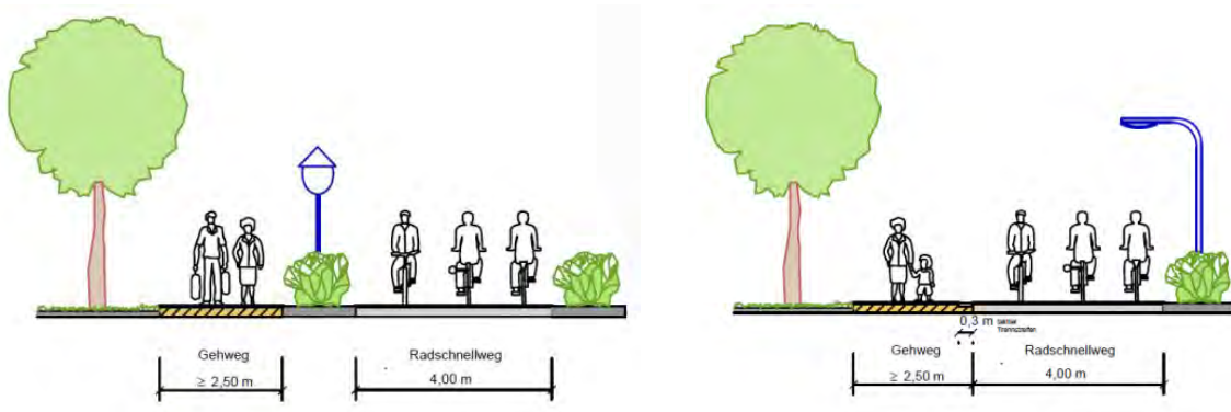
Abbildung 12: Musterquerschnitte für selbstständig geführte Verbindungen
